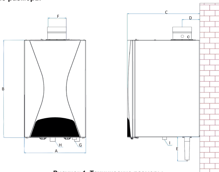
Рисунок 1. Технические размеры
